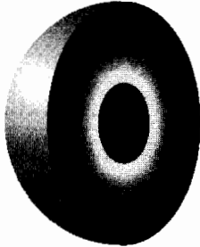
الشكل 5-8. تمثيل لبنية ذرّة الليثيوم. يوجد إلكترونان في قلب متراص، والإلكترون آخر في غلاف خارجي يحيط بالقلب.
